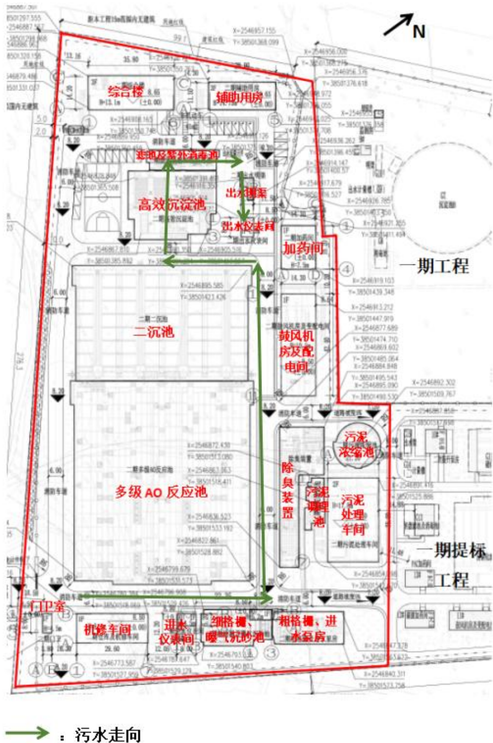
附图 9：各类废水走向图
