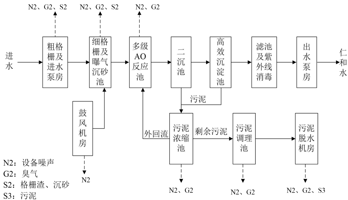
图 2.3-1 污水处理工艺流程图
