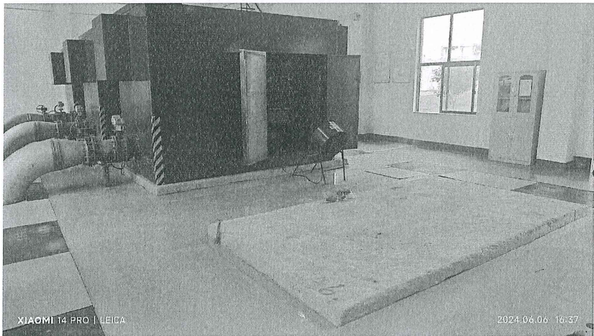
五、麻涌二期（风机基础尺寸为长 1.5m*宽 2.3m*高 0.3m）
