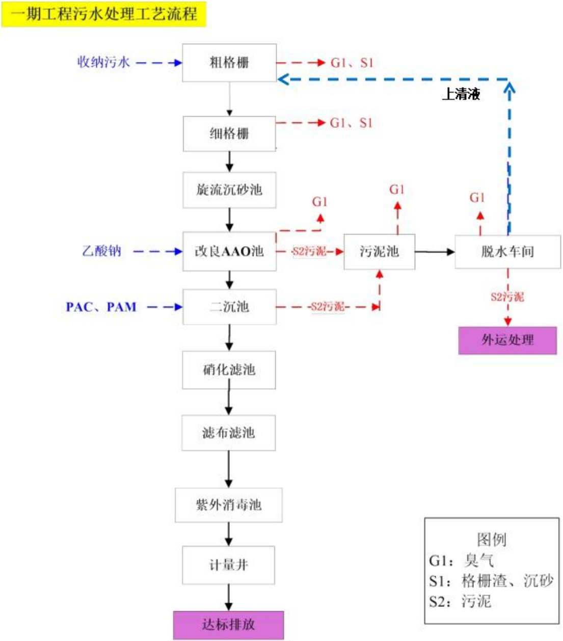
图 2.3-1 一期工程污水处理工艺流程图
