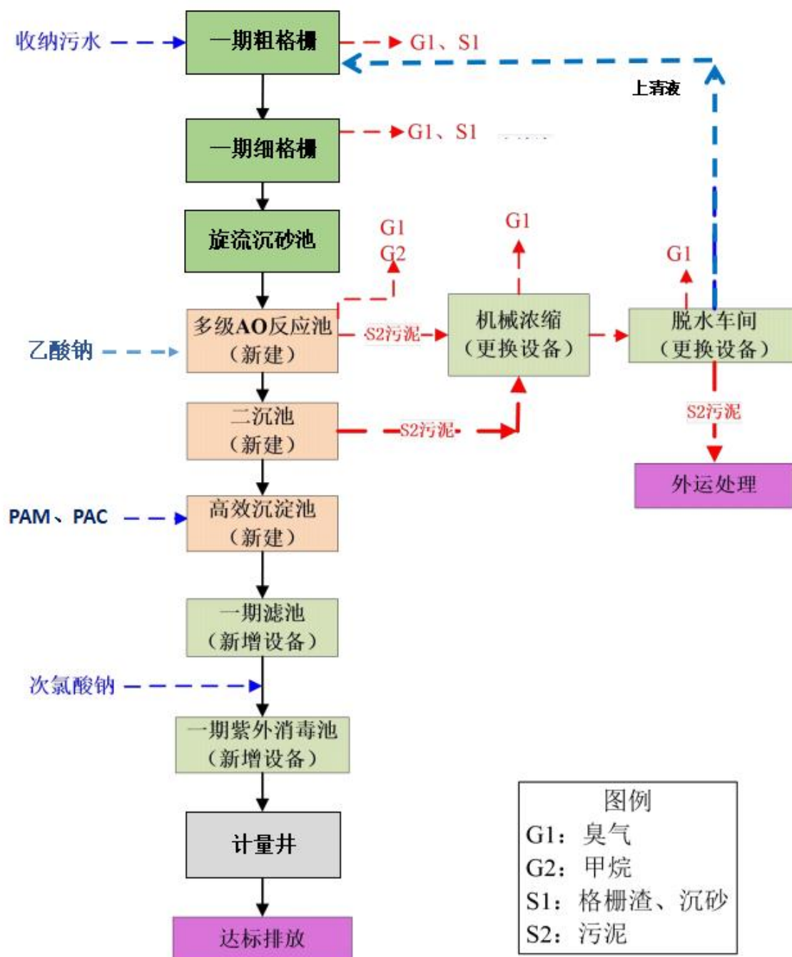
图 2.3-1 二期工程污水处理工艺流程图
