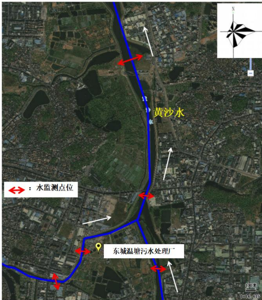
图6.7-1 废水监测布点图
