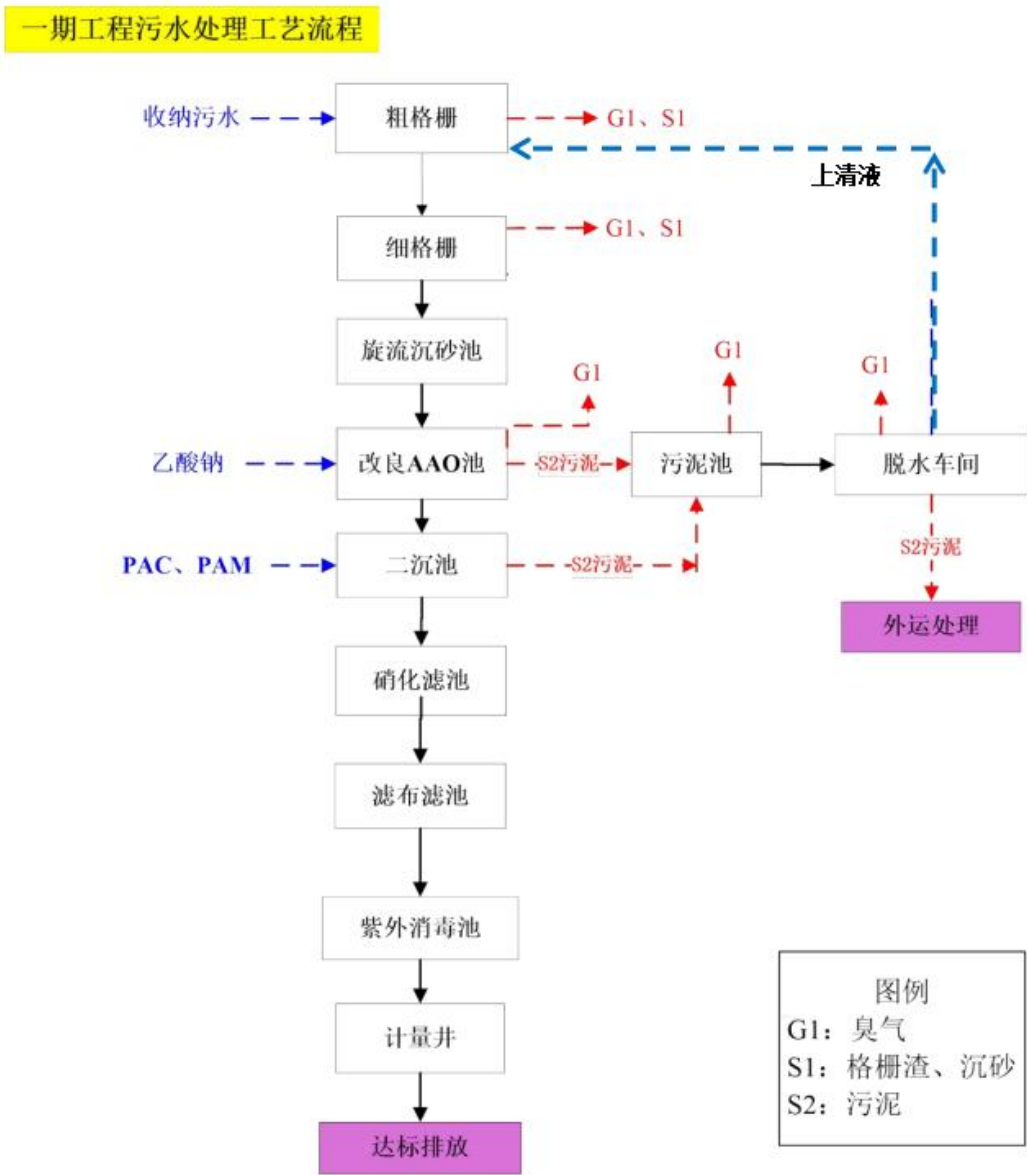
附图 11：污水处理工艺流程图
