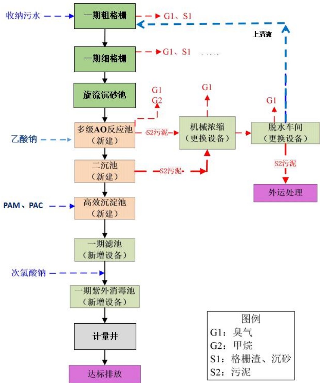
污水处理工艺流程图
