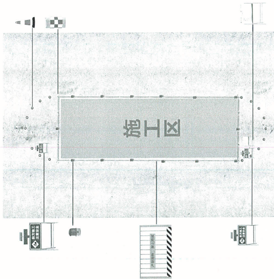
作业区域外围标准化配置示意图
