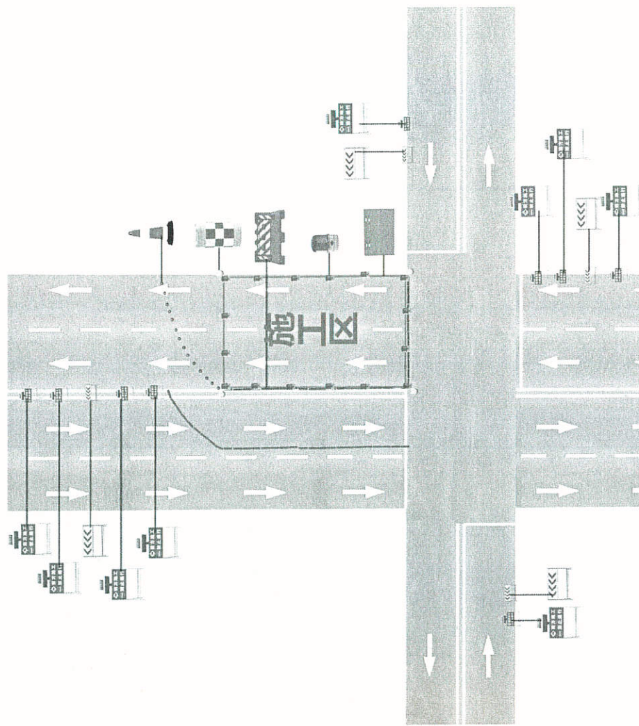
作业区域外围标准化配置示意图（十字路口单向占道施工）
