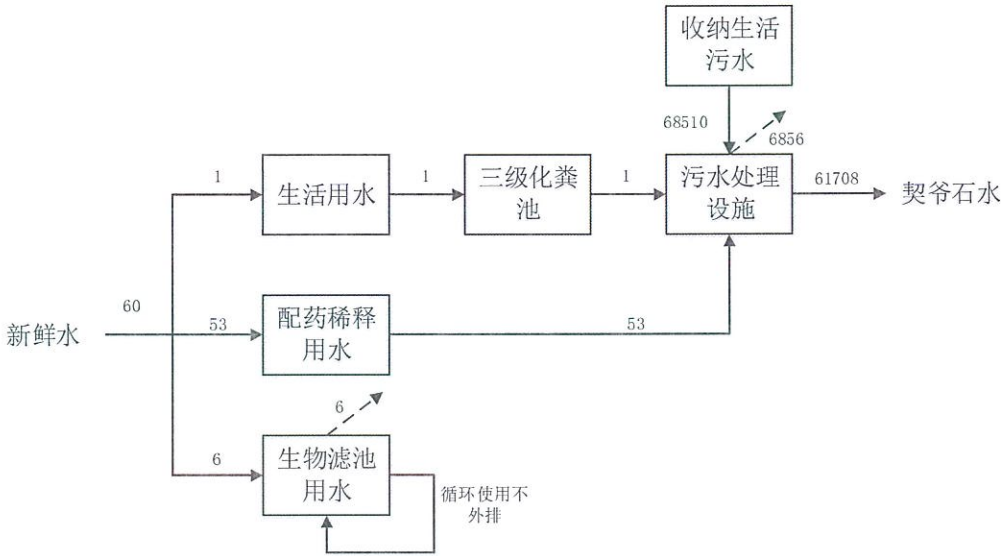
图 3.4-1 本项目验收监测期间（2024 年 9 月 18-19 日）水平衡图（单位：t）
