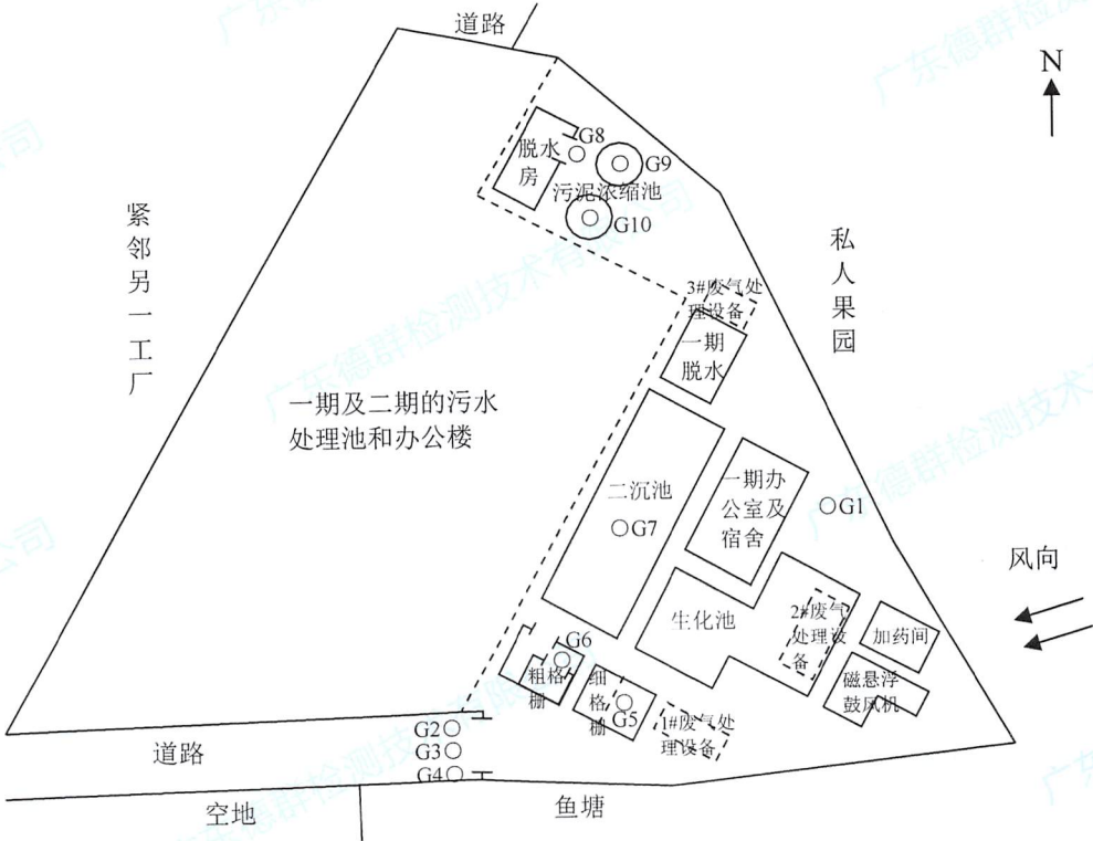
图 6 污水处理站恶臭污染物无组织排放监控点位示意图 (2024-09-12 第二次)
