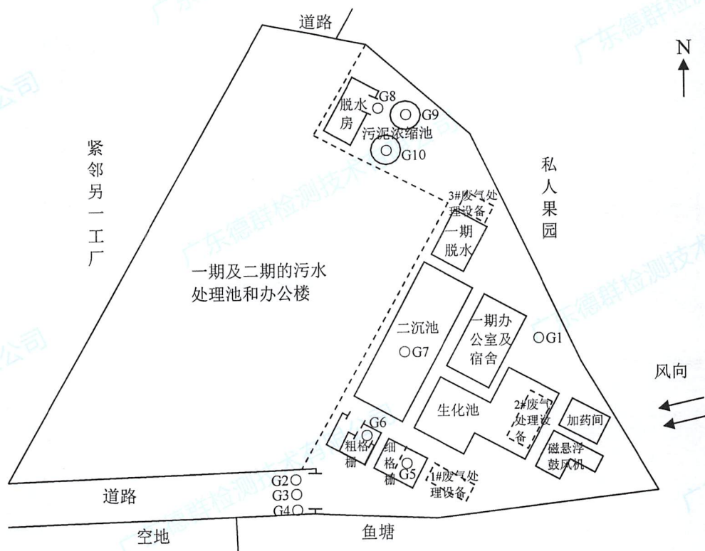
图2 污水处理站恶臭污染物无组织排放监控点位示意图 (2024-09-11 第二次)
