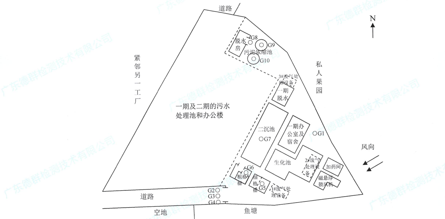
图 8 污水处理站恶臭污染物无组织排放监控点位示意图 (2024-09-12 第四次)
