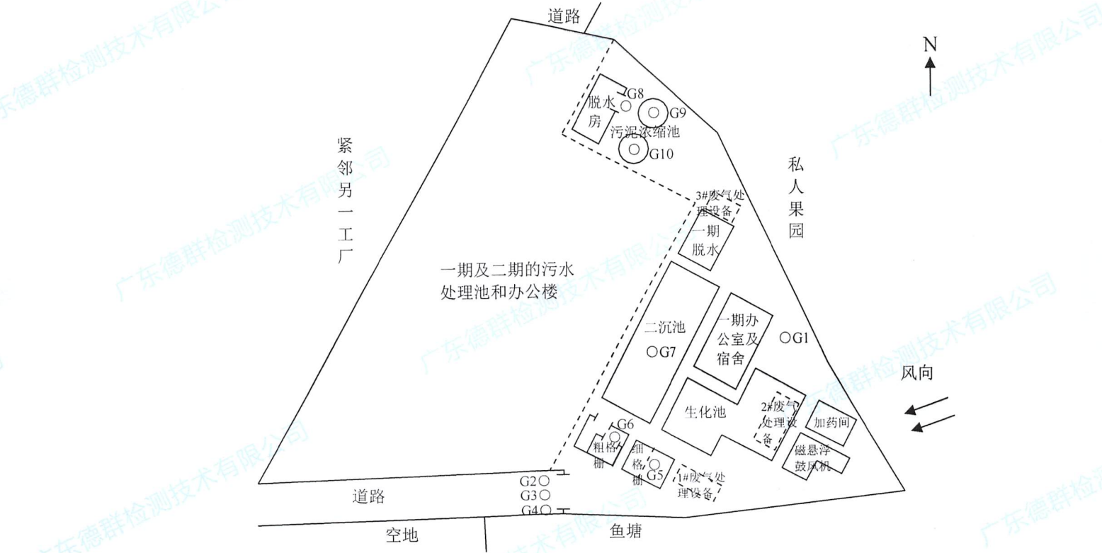
图 4 污水处理站恶臭污染物无组织排放监控点位示意图 (2024-09-11 第四次)
