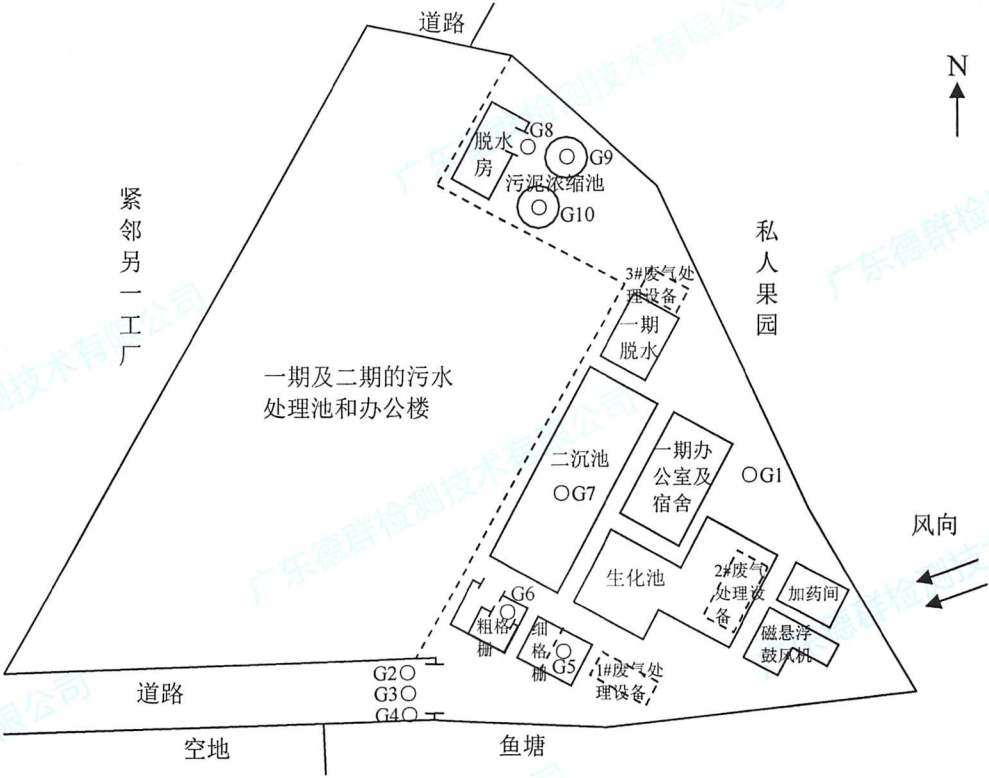
图 1 污水处理站恶臭污染物无组织排放监控点位示意图 (2024-09-11 第一次)
