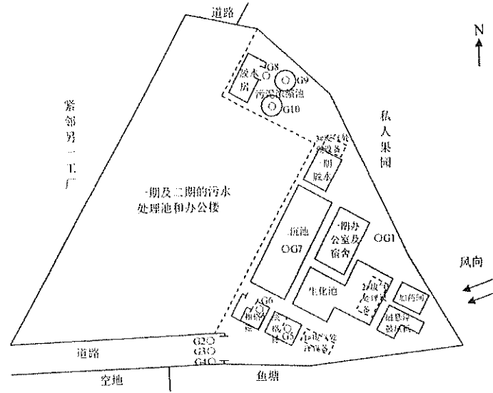
注: ○表示监控点位 图 5 污水处理站恶臭污染物无组织排放监控点位示意图 (2024-09-12 第一次)
