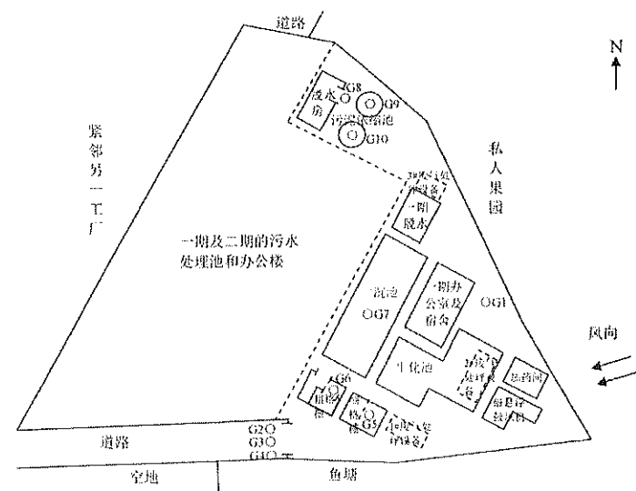
注: ○表示监控点位 图 6 污水处理站恶臭污染物无组织排放监控点位示意图 (2024-09-12 第二次)
