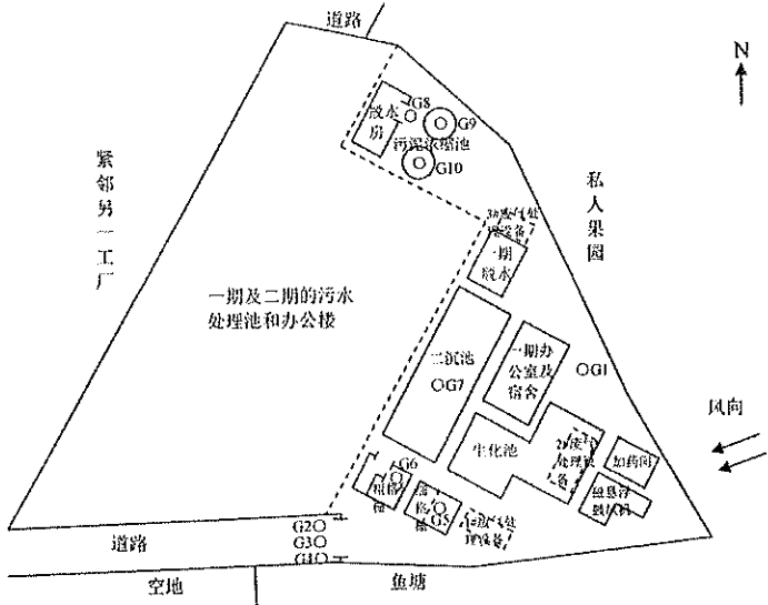
注: ○表示监控点位 图1 污水处理站恶臭污染物无组织排放监控点位示意图 (2024-09-11 第一次)
