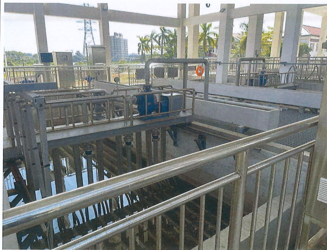
板框滤池
