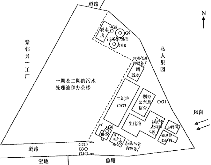
注：○表示监控点位 图 3 污水处理站恶臭污染物无组织排放监控点位示意图（2024-09-11 第三次）
