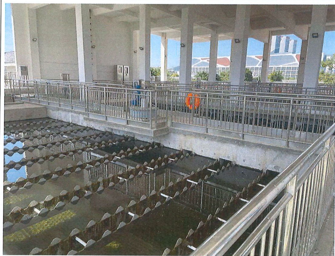
高效沉淀池
