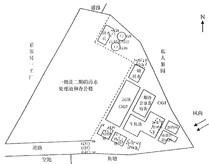
注: ○表示监控点位 图 7 污水处理站恶臭污染物无组织排放监控点位示意图 (2024-09-12 第三次)
