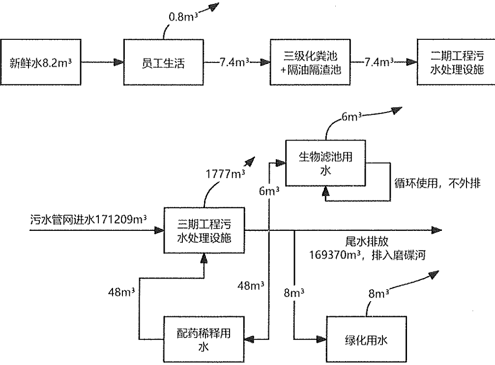
图3.4-1 本项目验收监测期间（2024年9月11-12日）两日水量水平衡图 3.5 生产工艺
