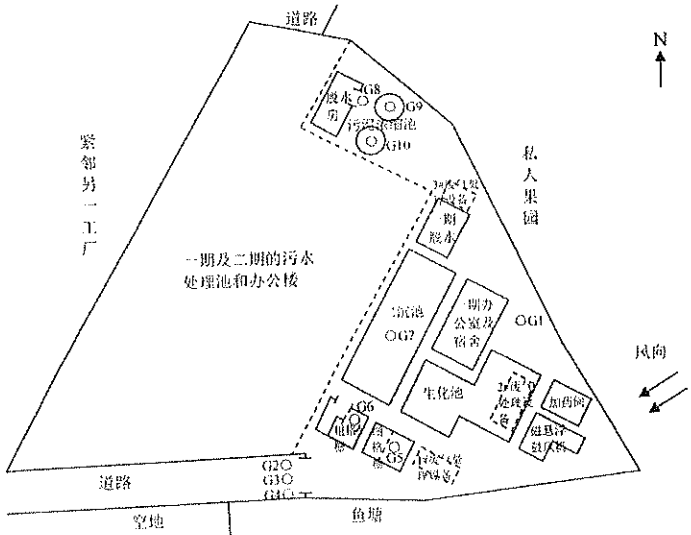
注: ○表示监控点位 图 4 污水处理站恶臭污染物无组织排放监控点位示意图 (2024-09-11 第四次)
