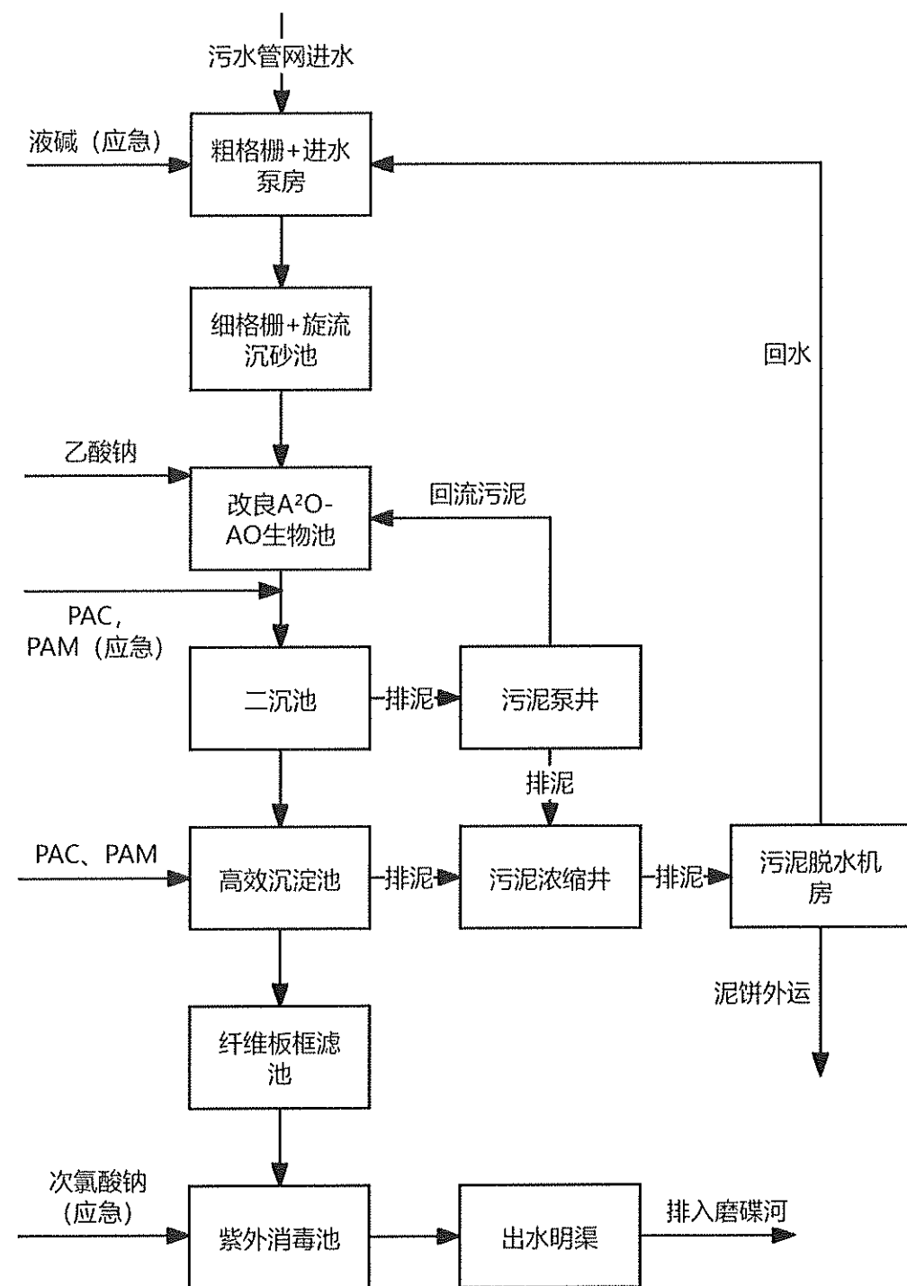
图3.5-1污水处理工艺流程图
